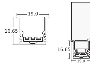
Sina 24V incastrata
