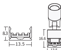
Sina 24V aplicata
