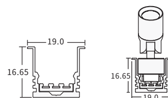
Sina 24V incastrata
